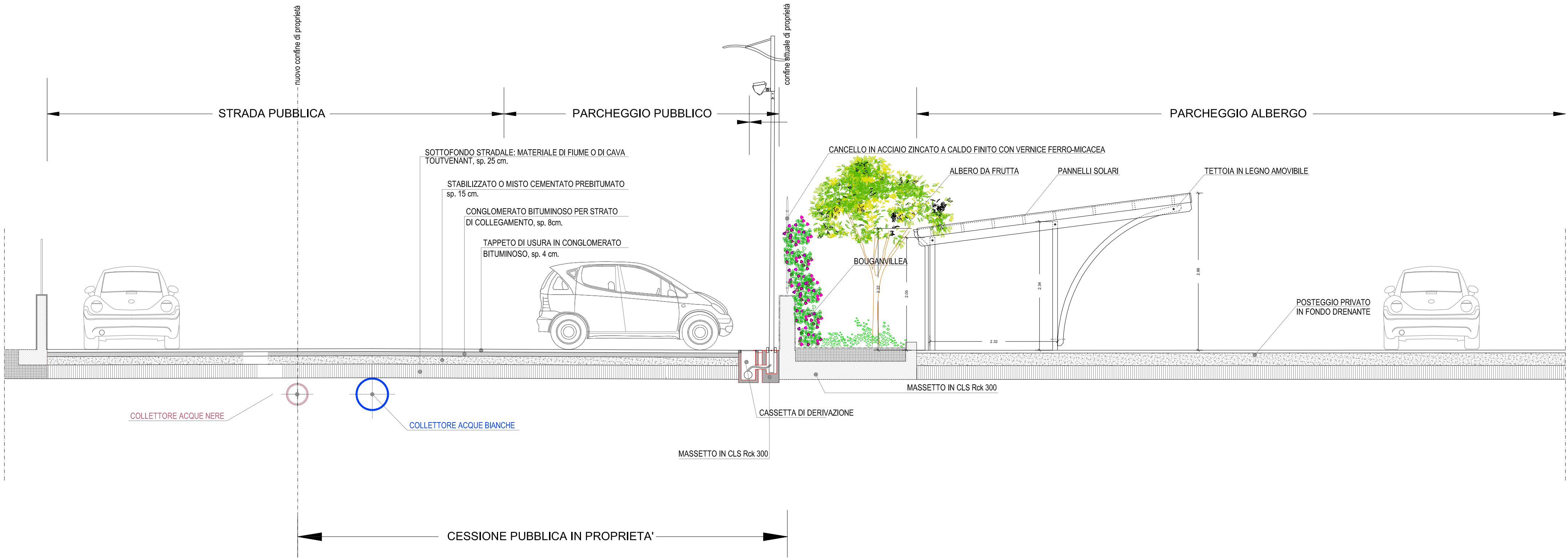
SEZIONE PARCHEGGIO PUBBLICO ED AD USO DELL'ALBERGO SCALA 1:50
