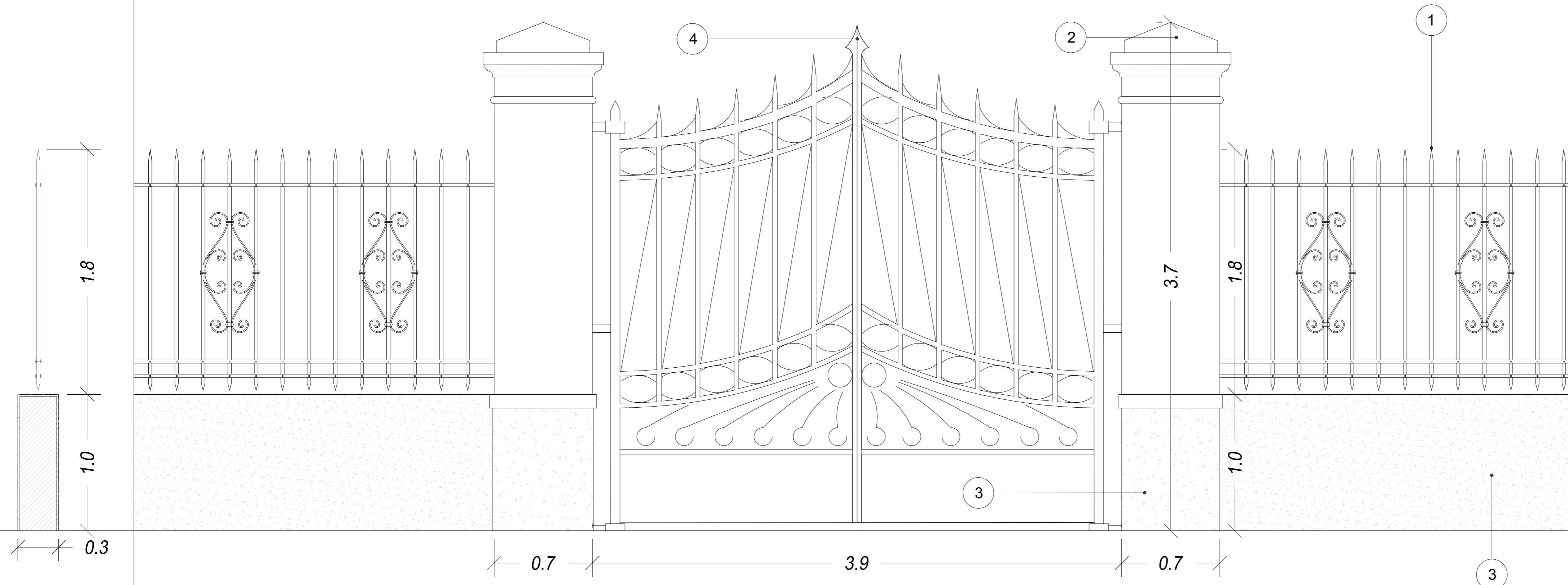
PARTICOLARE A
